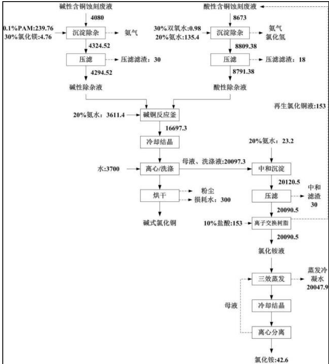
图 3.4-9 含铜蚀刻废液综合利用生产线水平衡图（单位： \text{m}^3/\text{a} ）
