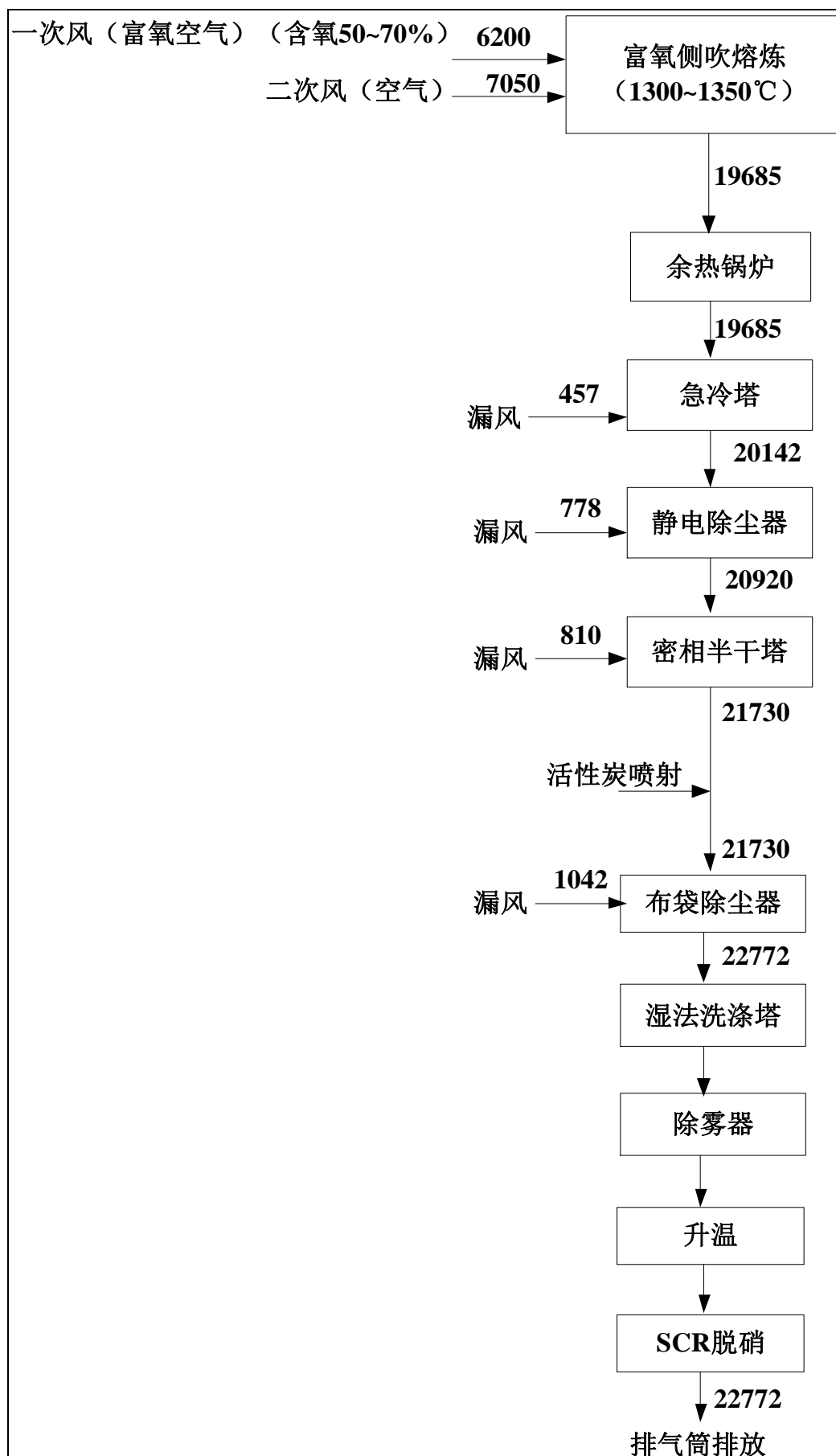
图 3.3-6 熔炼废气风量平衡图（单位：Nm 3 /h）
