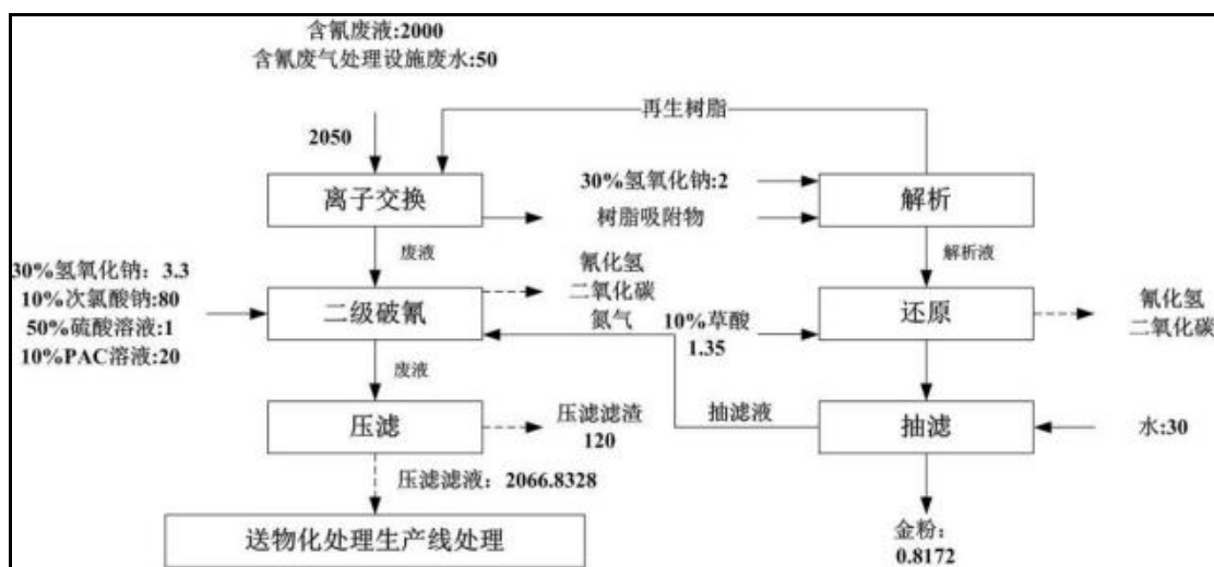
图 3.4-20 含氰废液综合利用生产线物料平衡图 (单位: m 3 /a)
