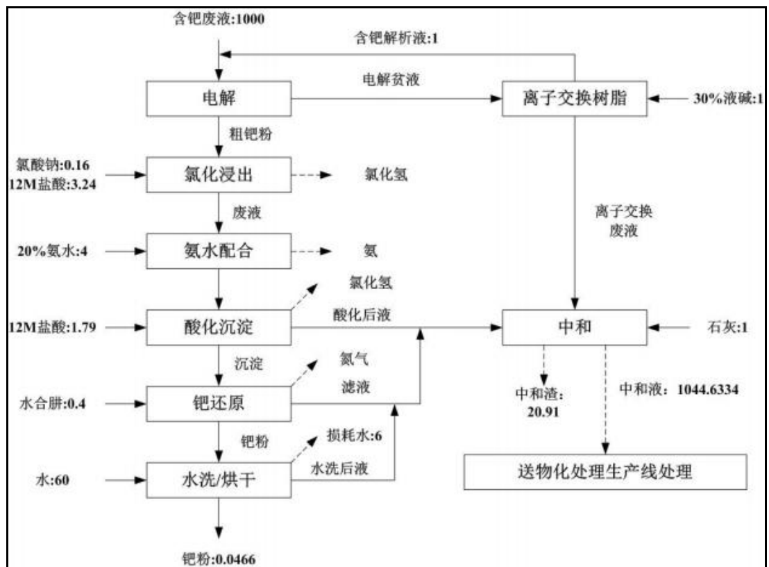
图 3.4-17 含钡废液综合利用生产线物料平衡图 (单位: m^3/a )
