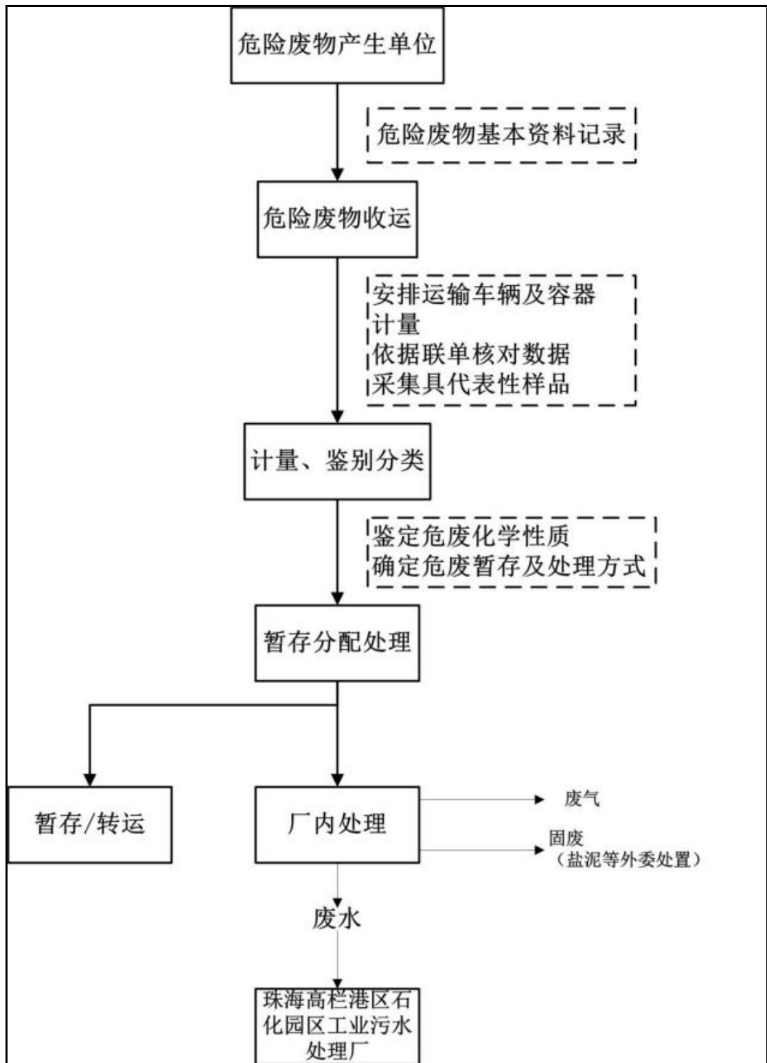
图 3.2-1 项目废物处理总体方案
