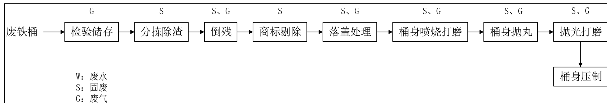
图 3.5-4 废铁桶处理工艺流程图
