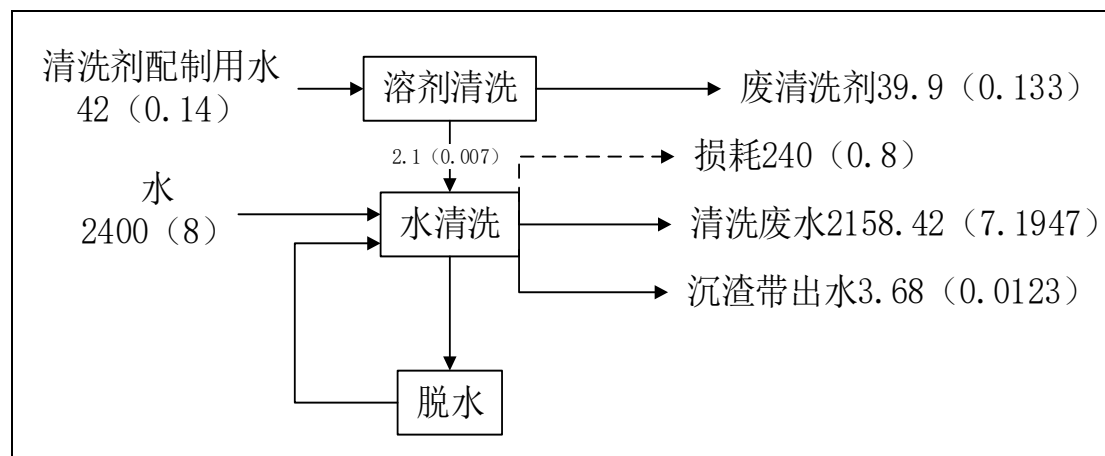
图 3.5-6 溶剂清洗回收生产线水平衡图（单位：t/a，括号内为 t/d）
