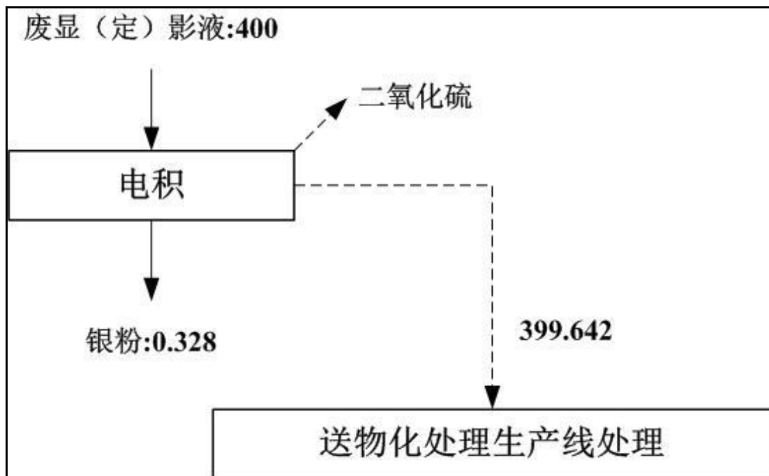
图 3.4-13 废显（定）影液综合利用生产线物料平衡图（单位：t/a）
