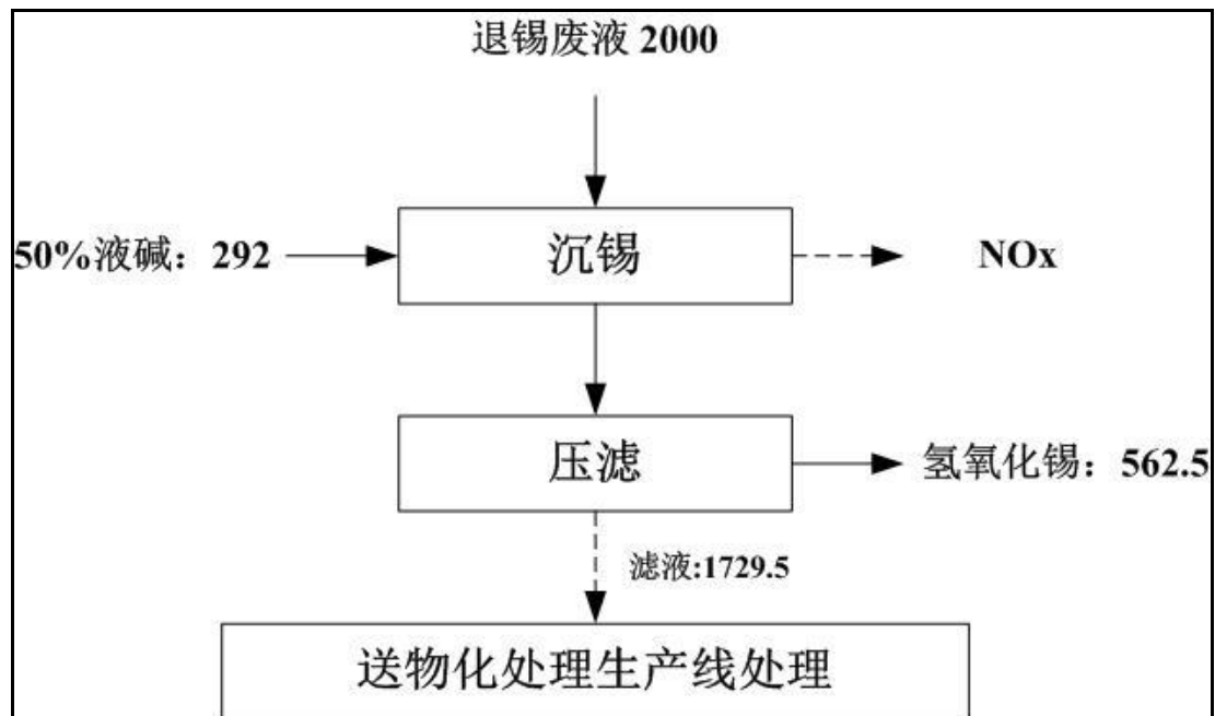
图 3.4-24 退锡废液综合利用生产线物料平衡图 (单位: t/a)
