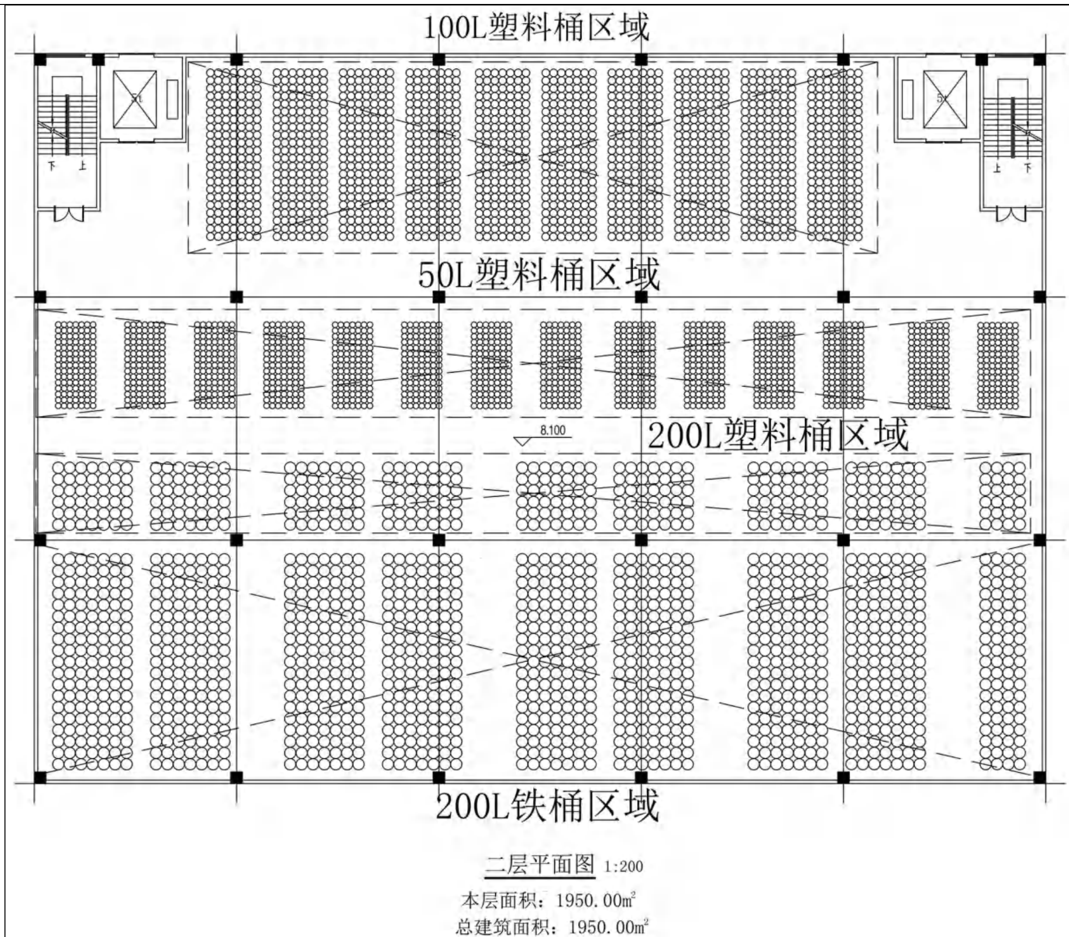
图 3.5-2 废包装桶车间二层平面布置图
