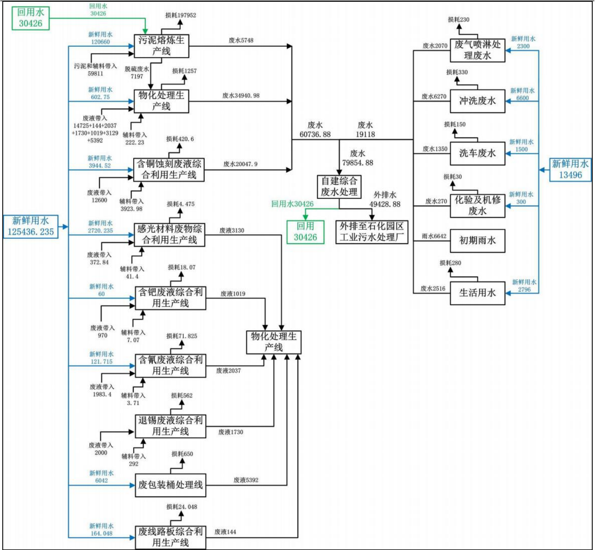
图 3.6-1 全厂水平衡图 (单位 m^3/a )
