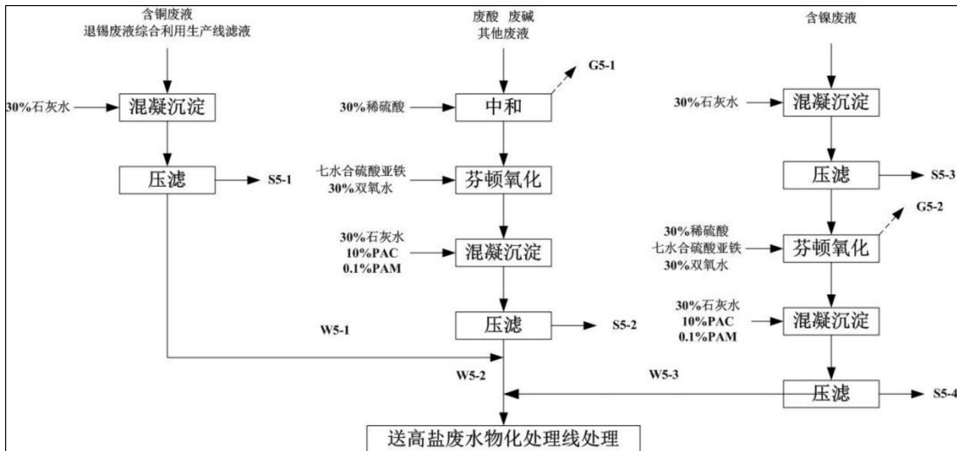
图 3.4-3 物化处理生产线工艺流程及产污环节图
