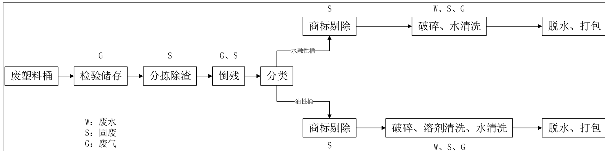
图 3.5-3 废塑料桶处理及产污环节图
