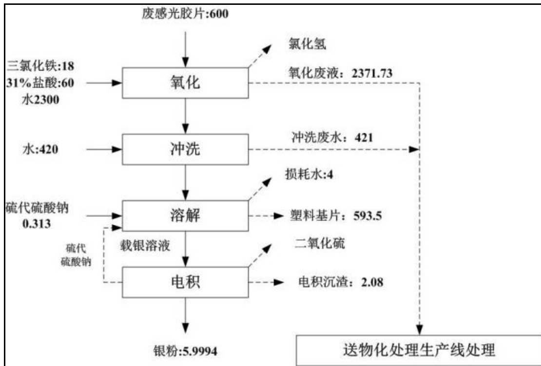
图 3.4-12 感废菲林胶片综合利用生产线物料平衡图（单位：t/a）
