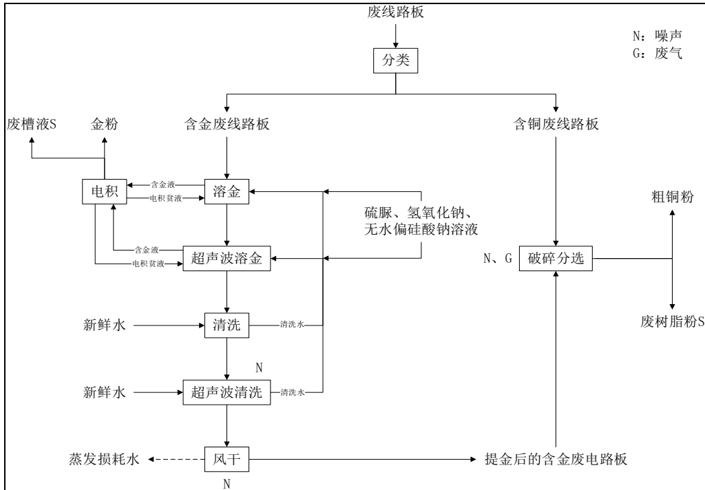
图 3.5-9 废电路板综合利用工艺流程图
