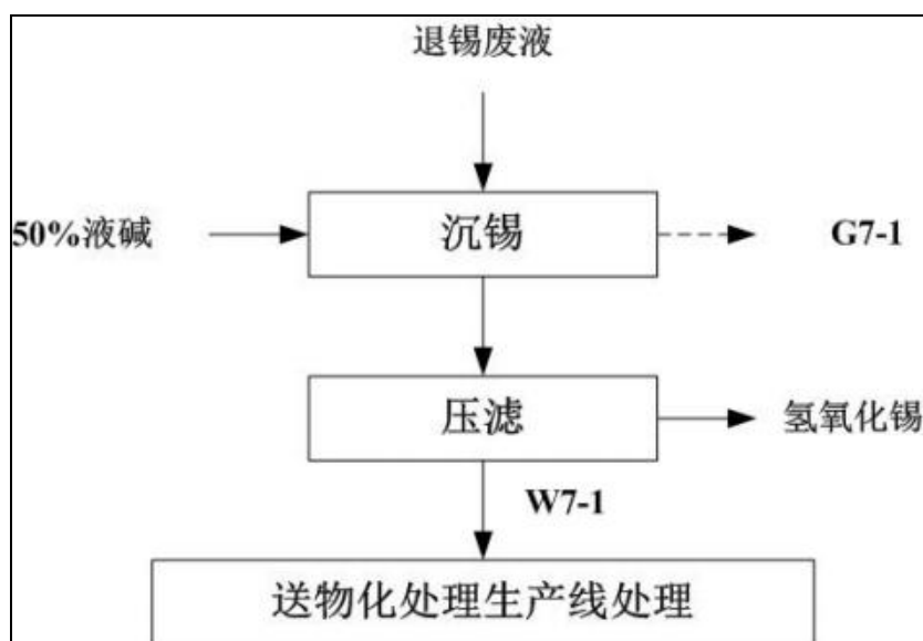
图 3.4-22 退锡废液综合利用生产线工艺流程及产污环节图
