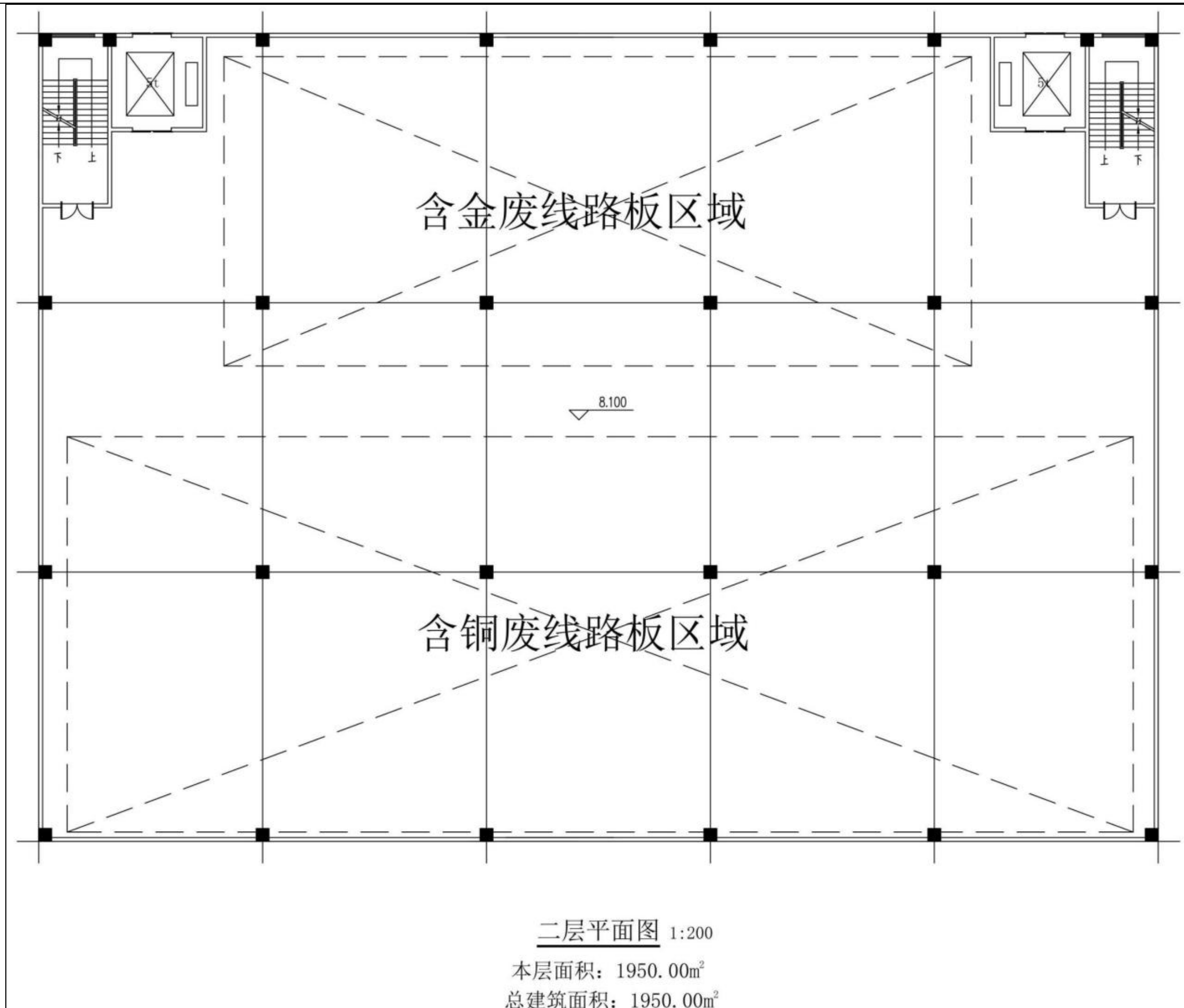
图 3.5-8 废线路板车间二层平面布置图
