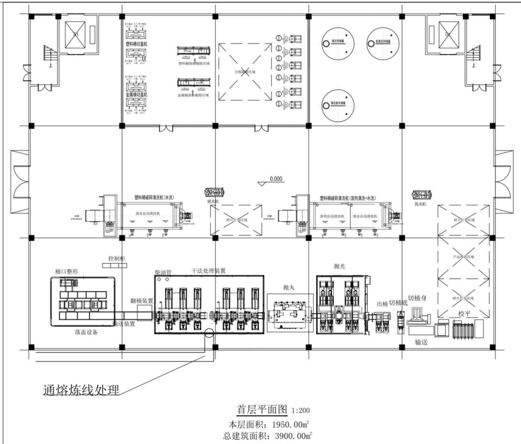
图 3.5-1 废包装桶车间首层平面布置图
