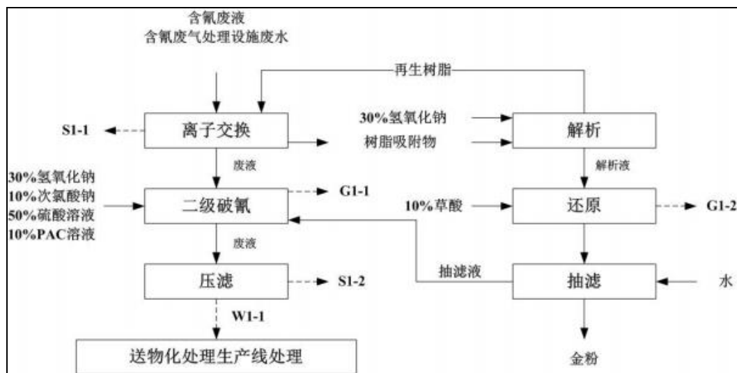
图 3.4-19 含氰废液综合利用生产线工艺流程及产污环节图
