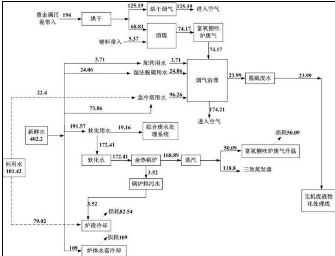
图 3.3-7 污泥熔炼生产线水平衡图 (单位: m³/d)
