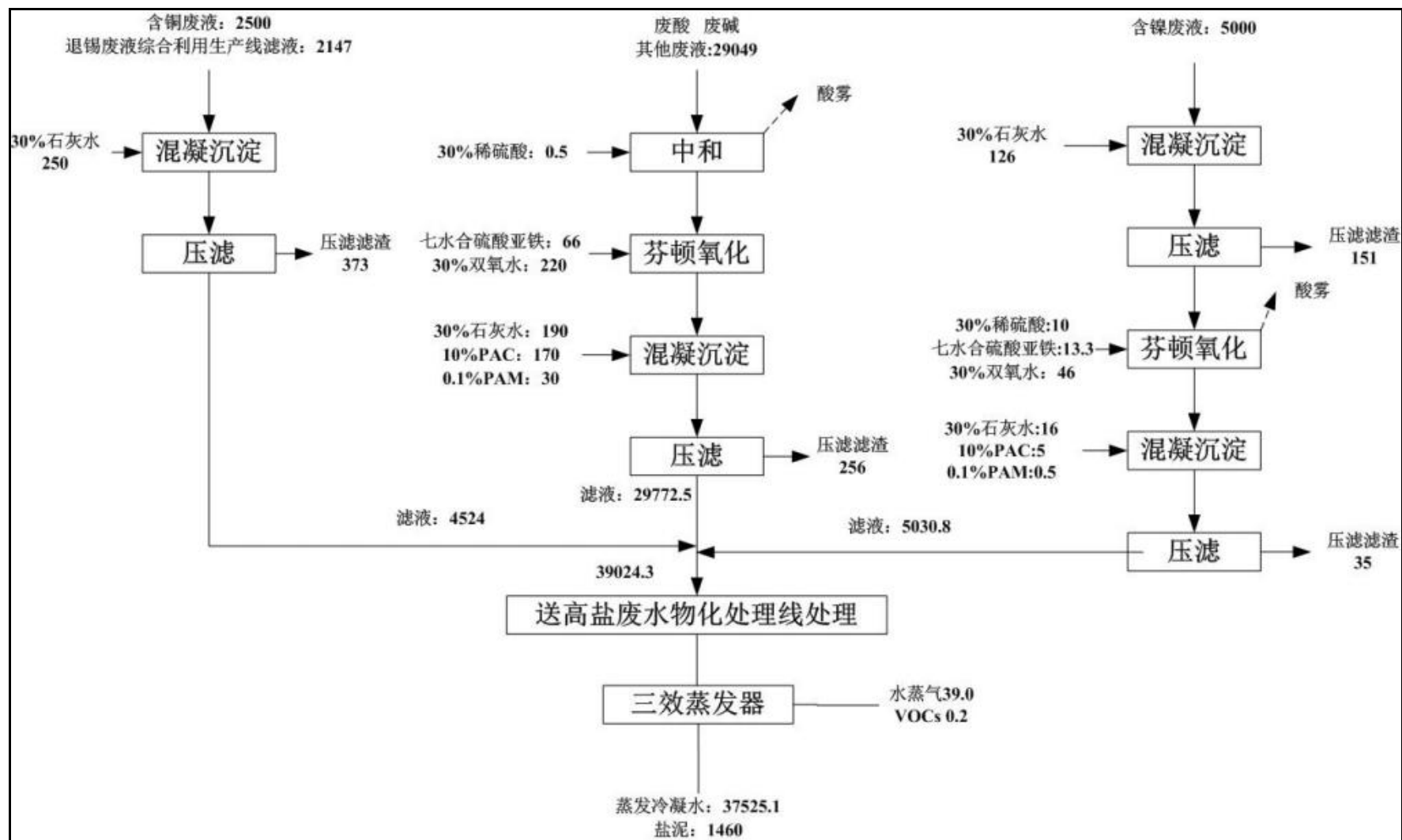
图 3.4-5 物化处理生产线物料平衡图
