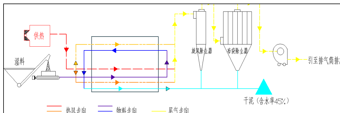
图 3.3-4 三级多回路烘干机示意图
