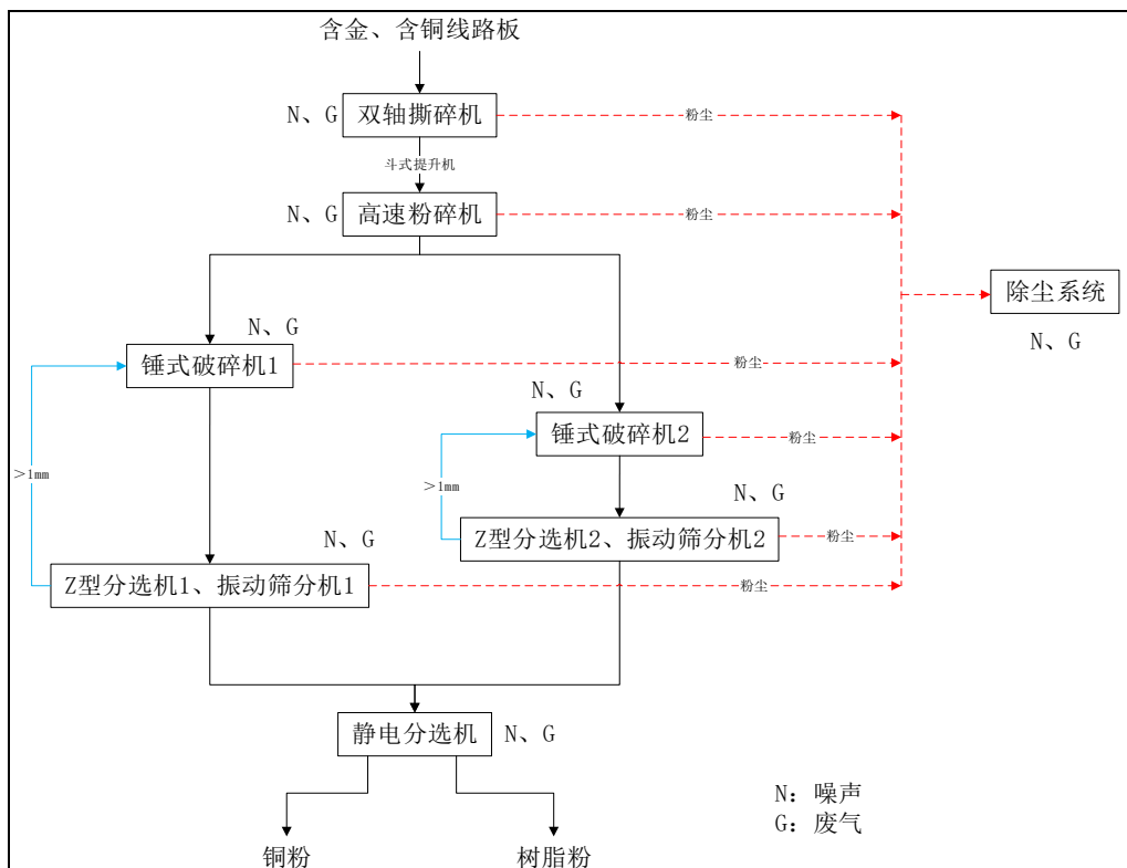
图 3.5-10 废线路板破碎分选工序工艺流程图
