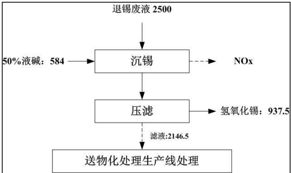
图 3.4-23 退锡废液综合利用生产线物料平衡图 单位: t/a
