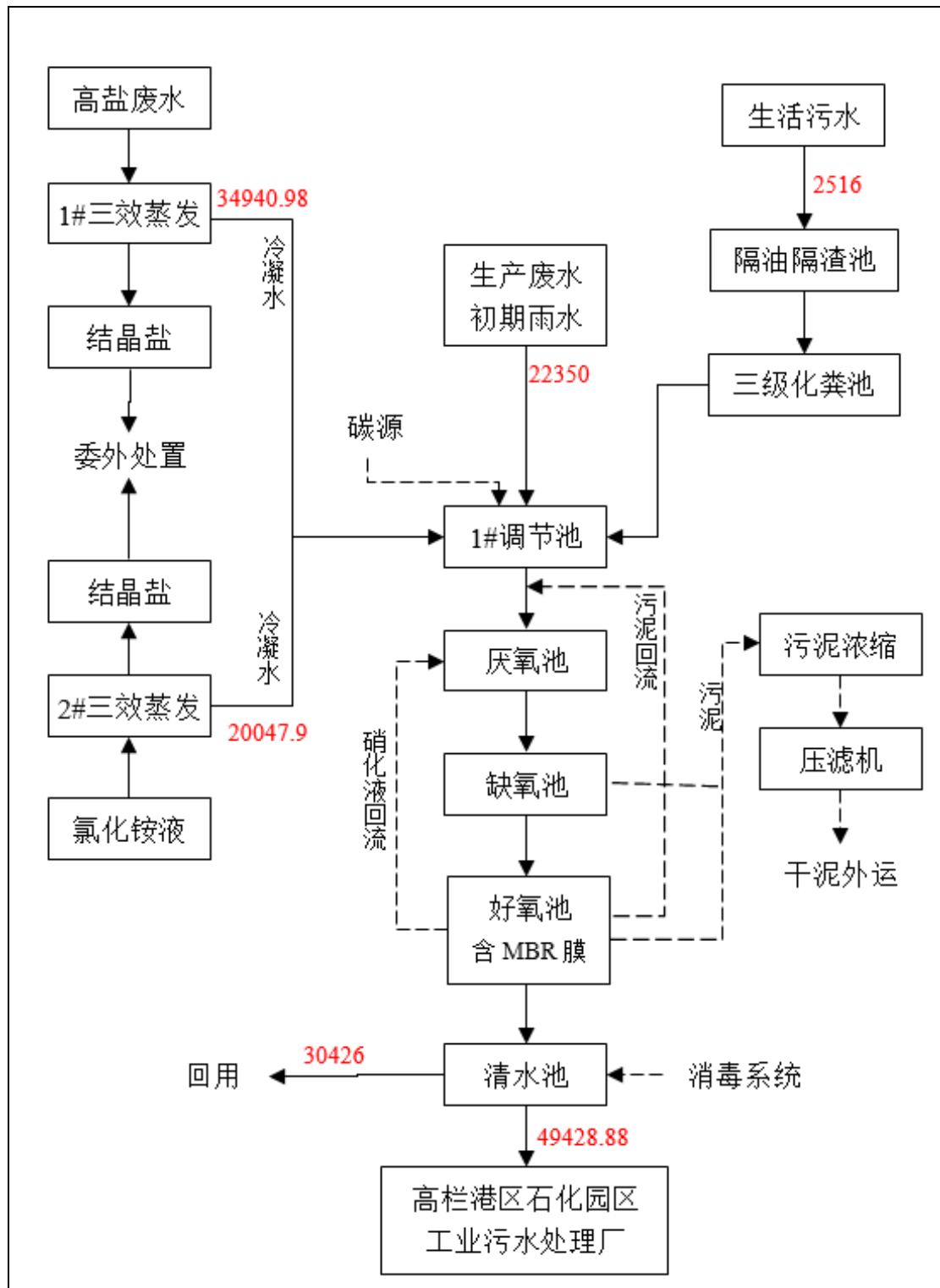
图 6.2-1 本项目废水处理工艺流程图
