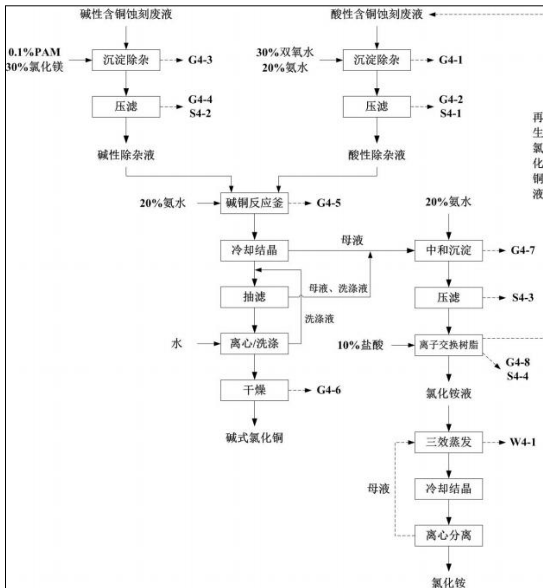
图 3.4-7 含铜蚀刻废液综合利用生产线工艺流程及产污环节图
