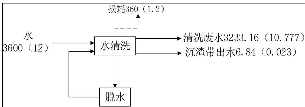
图 3.5-5 水清洗回收生产线水平衡图（单位：t/a，括号内为 t/d）
