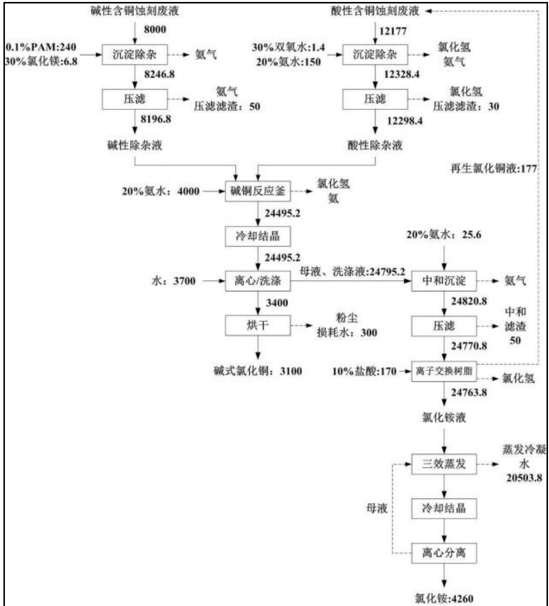
图 3.4-8 含铜蚀刻废液综合利用生产线物料平衡图（单位：t/a）
