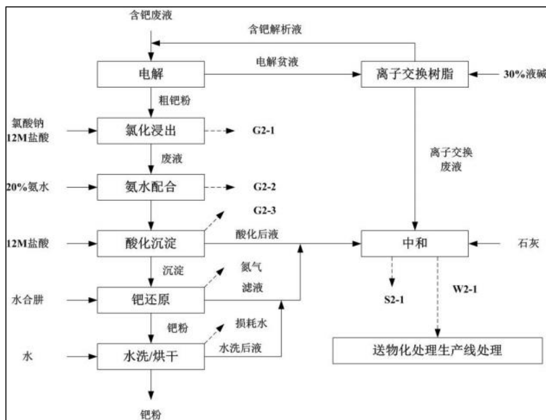
图 3.4-16 含钡废液综合利用生产线工艺流程及产污环节图
