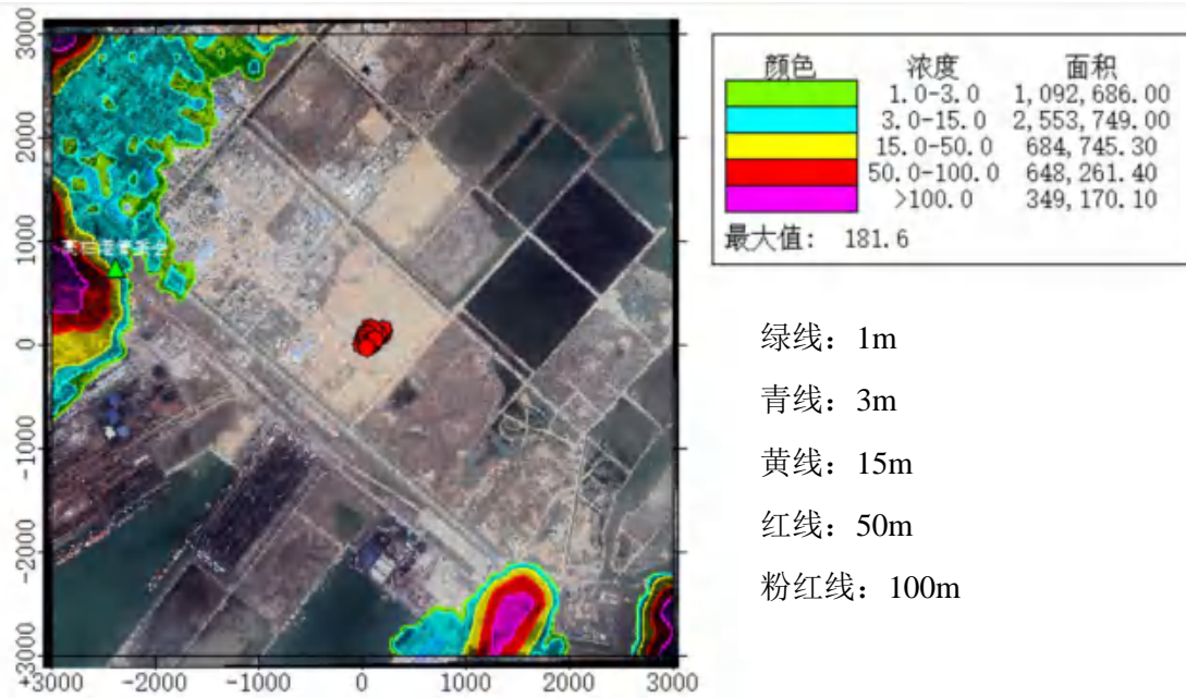
图 5.1-7 预测区域地形特征图
