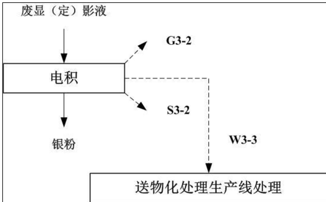
图 3.4-11 废显（定）影液综合利用生产线工艺流程及产污节点图
