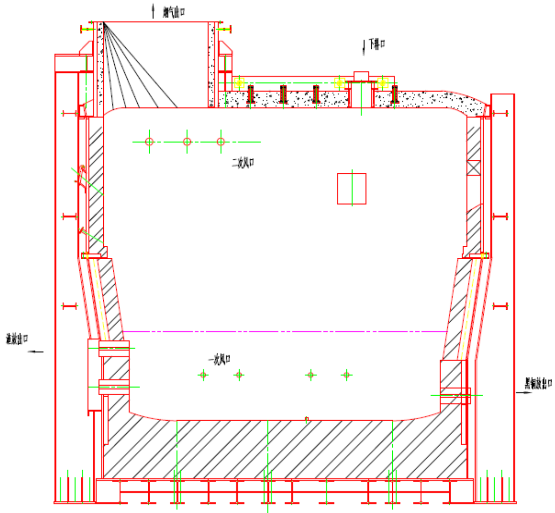
图 3.3-5 熔炼生产线富氧侧吹浸没燃烧炉结构示意图
