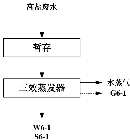
图 3.4-4 高盐废水物化处理线工艺流程及产污环节图
