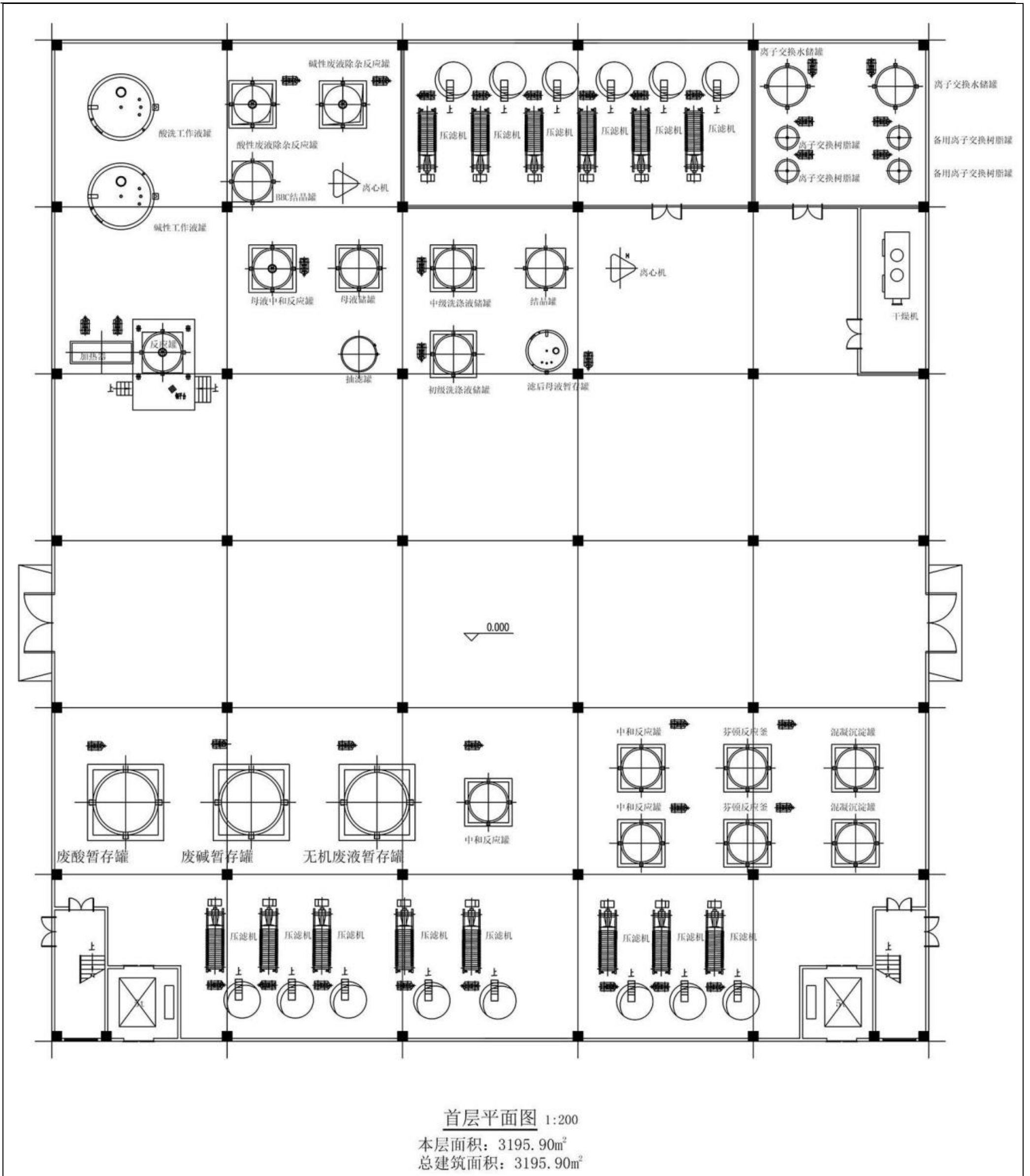
图 3.4-1 物化车间平面布置图 (一层)
