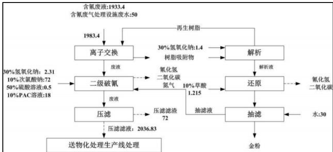
图 3.4-21 含氰废液综合利用生产线水平衡图 (单位: \text{m}^3/\text{a} )
