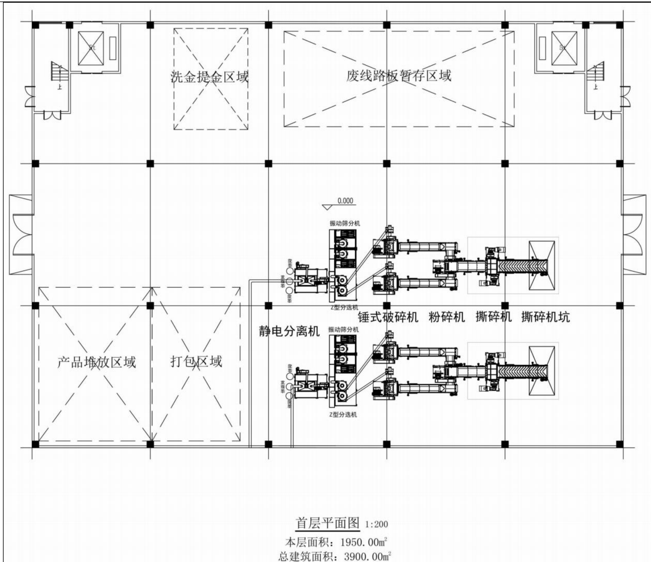
图 3.5-7 废线路板车间首层平面布置图
