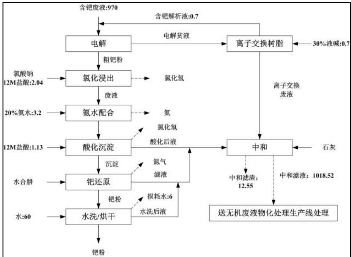
图 3.4-18 含钡废液综合利用生产线水平衡图（单位： \text{m}^3/\text{a} ）
