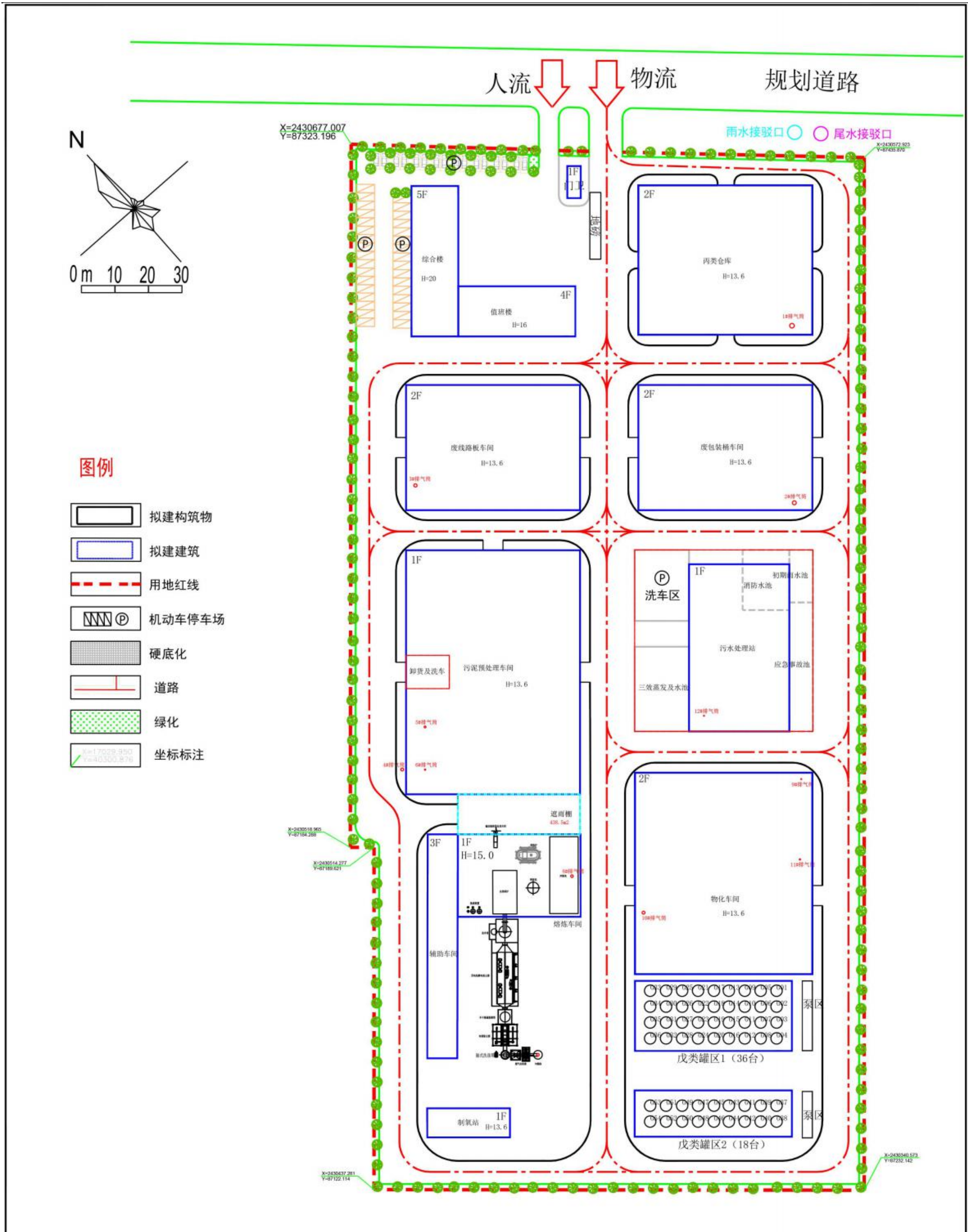
图 3.1-4 项目总平面布置图
