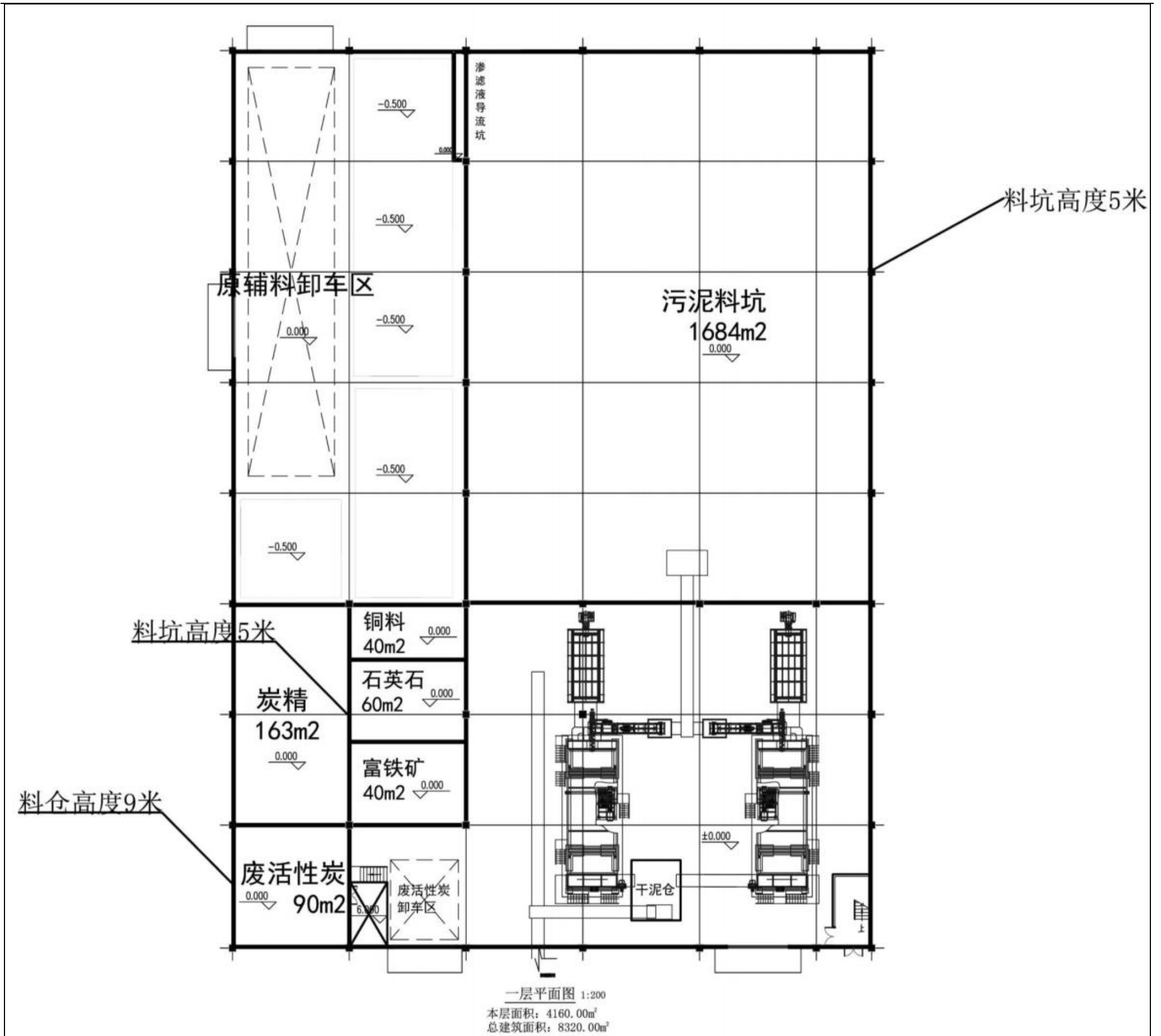
图 3.3-1 熔炼生产线（污泥预处理车间）平面布置图
