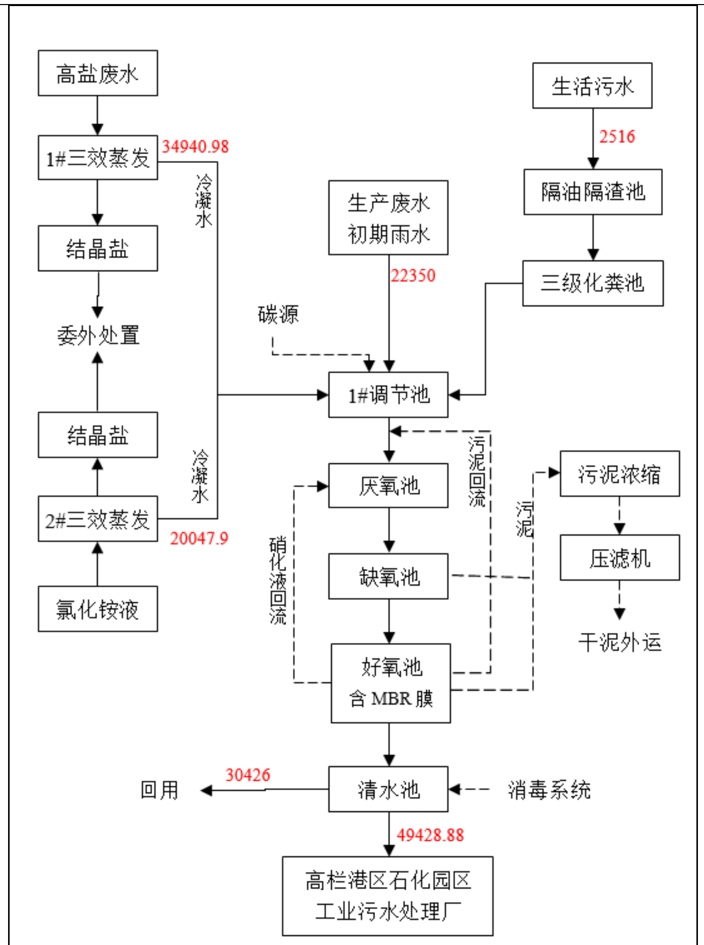
图 3.1-5 废水处理工艺流程图
