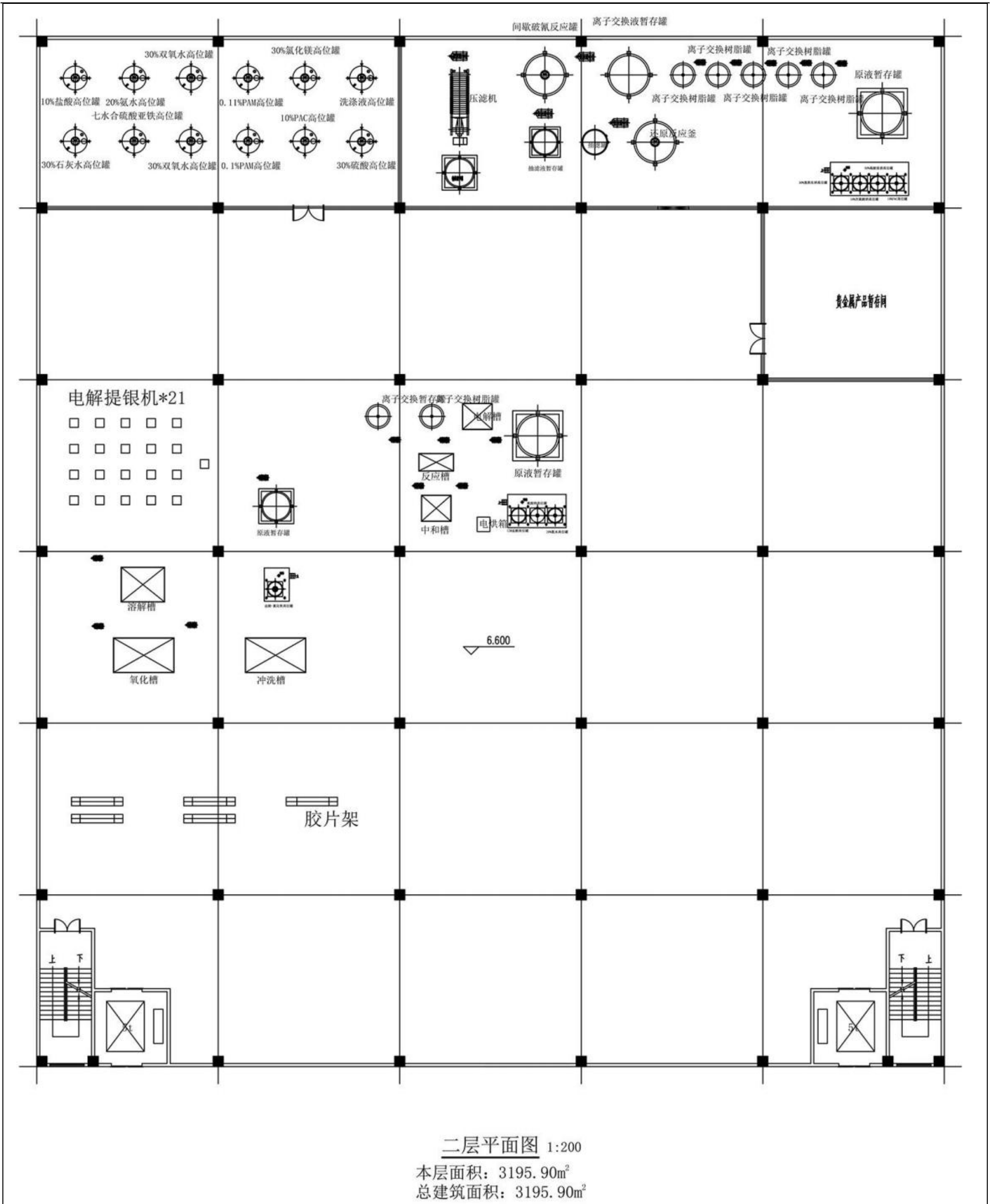
图 3.4-2 物化车间平面布置图（二层）
