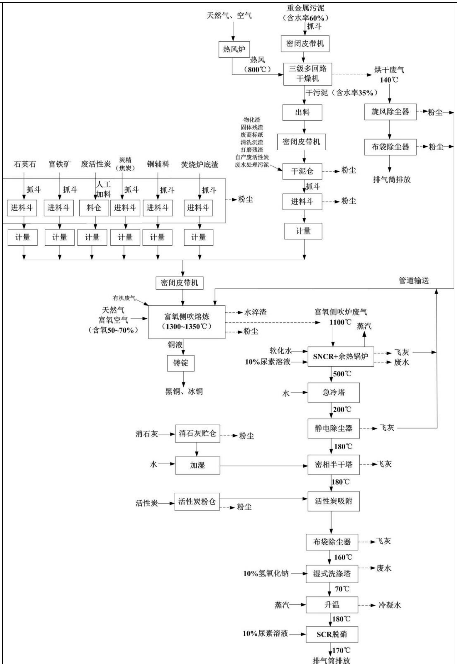
图 3.3-3 污泥熔炼车间工艺流程图及产污环节
