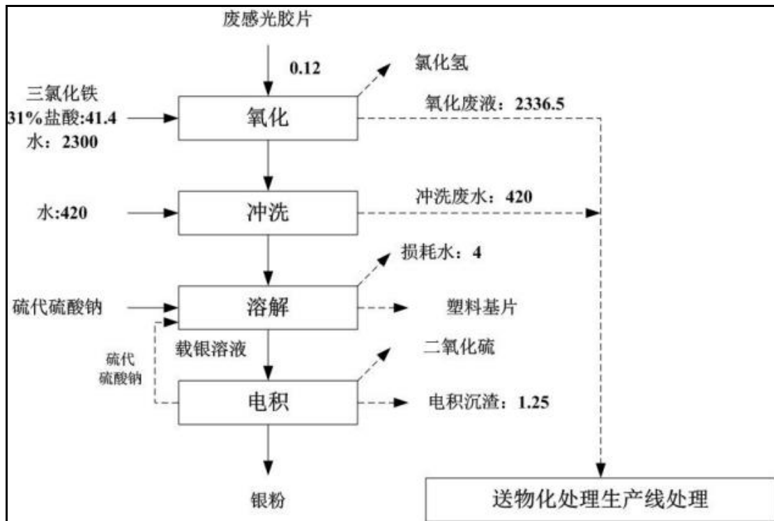
图 3.4-14 感废菲林胶片综合利用生产线水平衡图 (单位: \text{m}^3/\text{a} )
