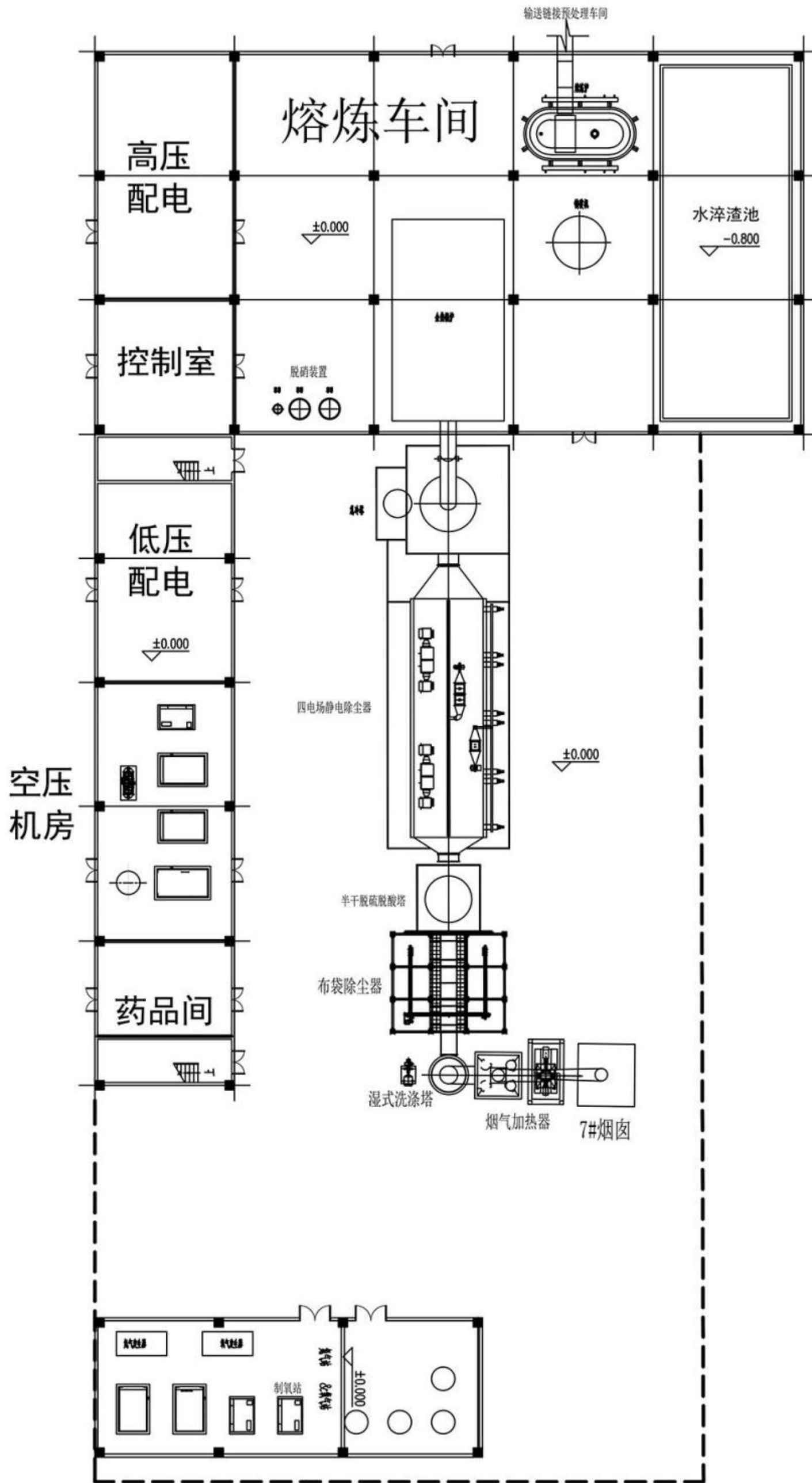
一层平面图 1:200 总占地面积: 3462m 2 总建筑面积: 2710.30m 2
