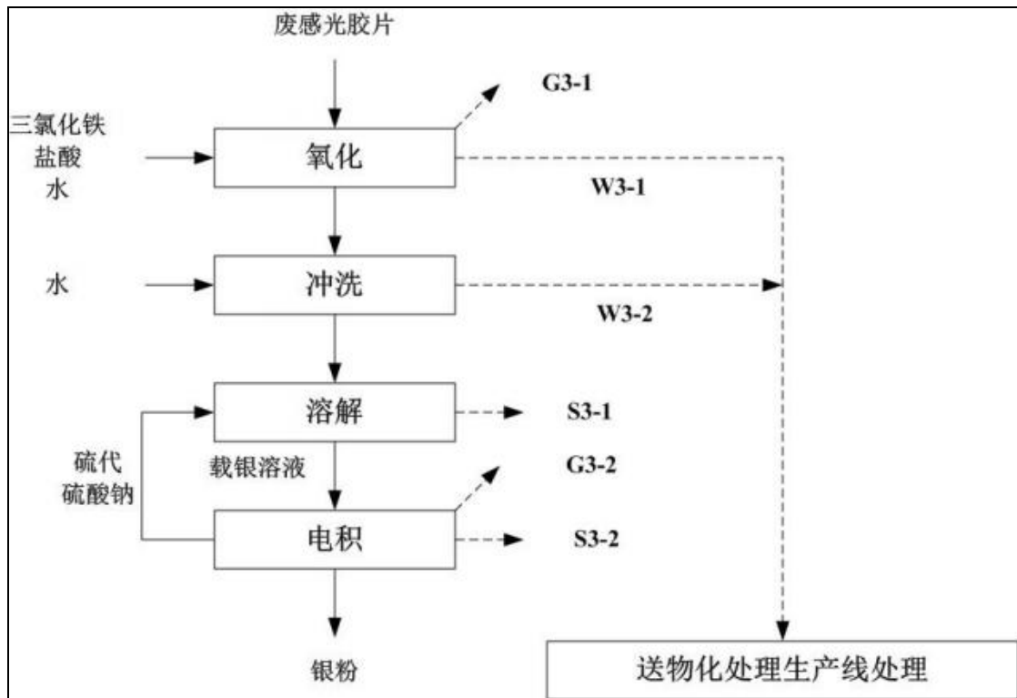
图 3.4-10 废菲林胶片综合利用生产线工艺流程及产污节点图
