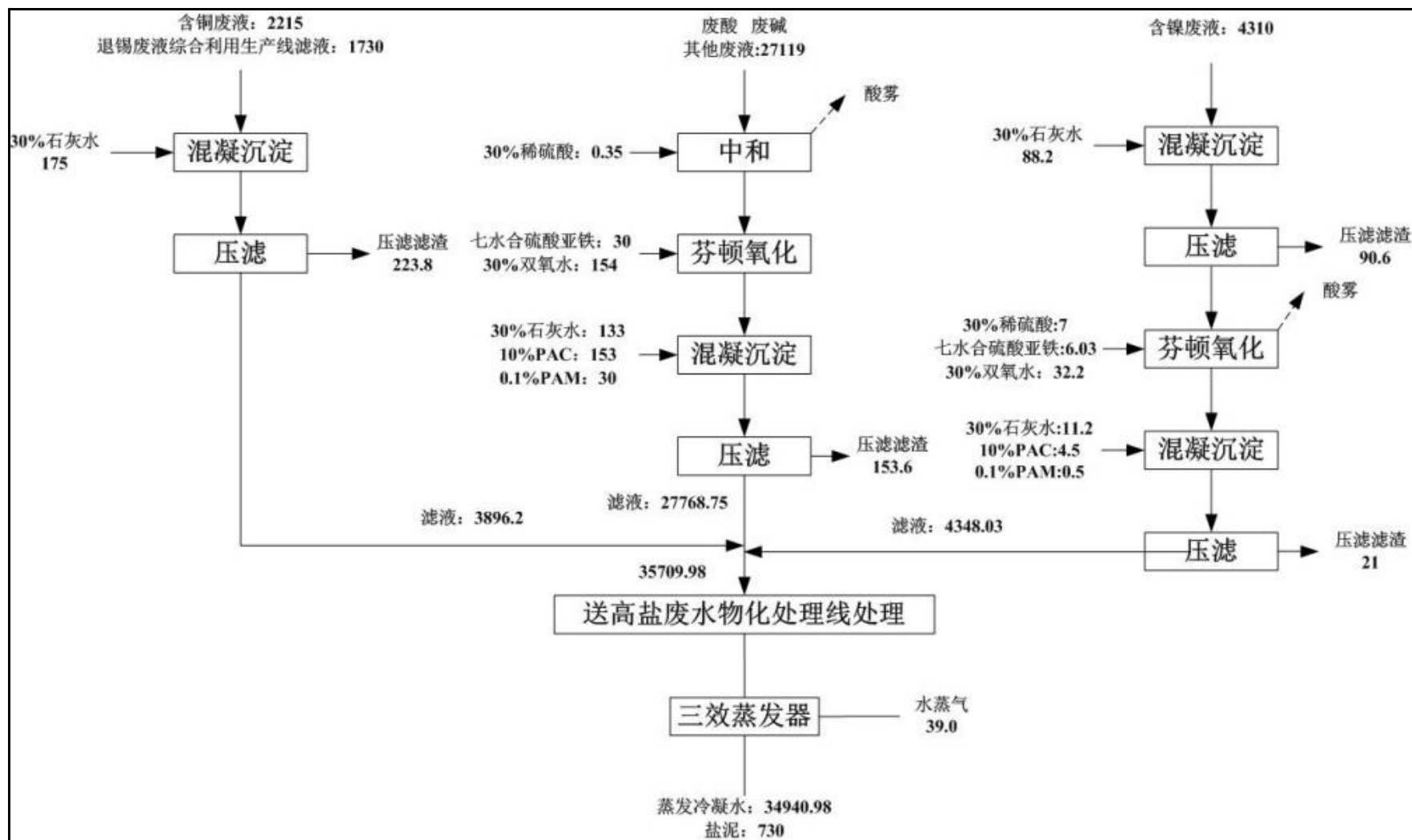
图 3.4-6 物化处理生产线水平衡图 (单位: \text{m}^3/\text{a} )
